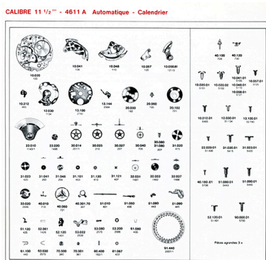
Calibre 11 1/2'' - 4611- A Automatique Calendrier [éclaté des fournitures], 1973. IVR43_20162500140NUC2A
