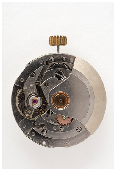
Mouvement FE 4612, vu côté ponts. Phot. Sonia Dourlot IVR43_20152502556NUC4A
