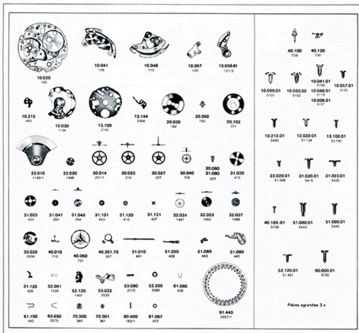
Calibre 11 1/2''' - 4611-A Automatique Calendrier [éclaté des fournitures], 1973.
